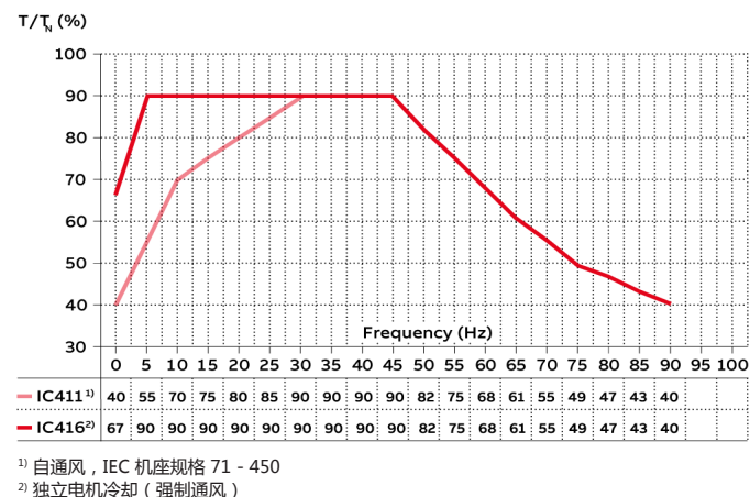
图 7. 增安型电机 Ex ec/ Ex nA，铸铁和铝质粉尘防爆型电机 Ex t/Ex tD T125°C；电机标称频率为 50/60 Hz
