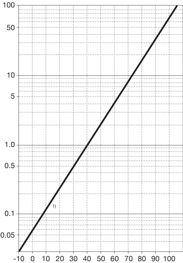
图 1. 图中所示为绝缘电阻与温度的关系以及如何将测得的绝缘电阻按 40°C 纠正。
