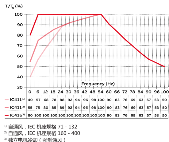
图 6. 隔爆型电机 Ex d/Ex db / Ex de/Ex db eb T4，铸铁粉尘防爆型电机 Ex t T150°C；电机标称频率为 50/60 Hz
