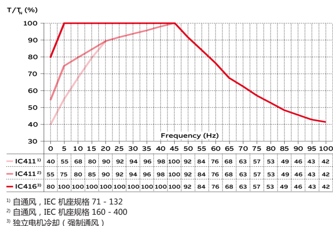
图 6. 隔爆型电机 Ex d/Ex db / Ex de/Ex db eb T4，铸铁粉尘防爆型电机 Ex t T150°C；电机标称频率为 50/60 Hz
